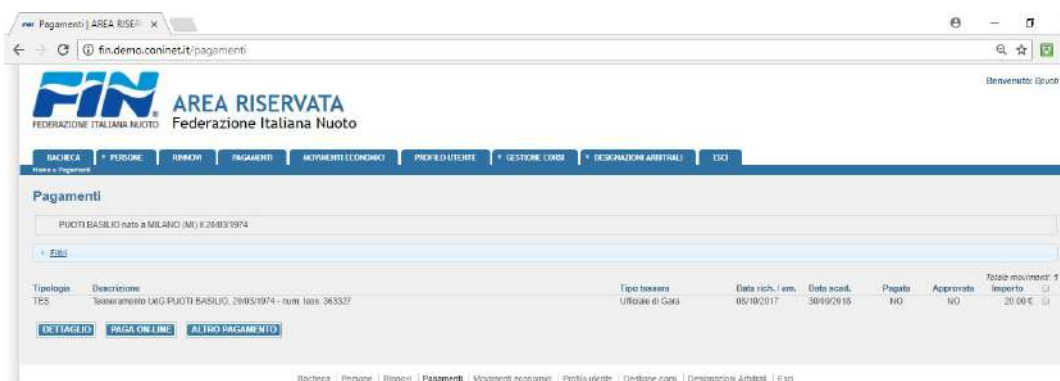
Figura 18: maschera pagamenti
