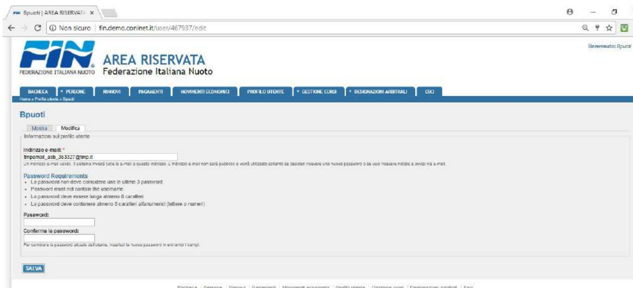
Figura 33: modifica password
