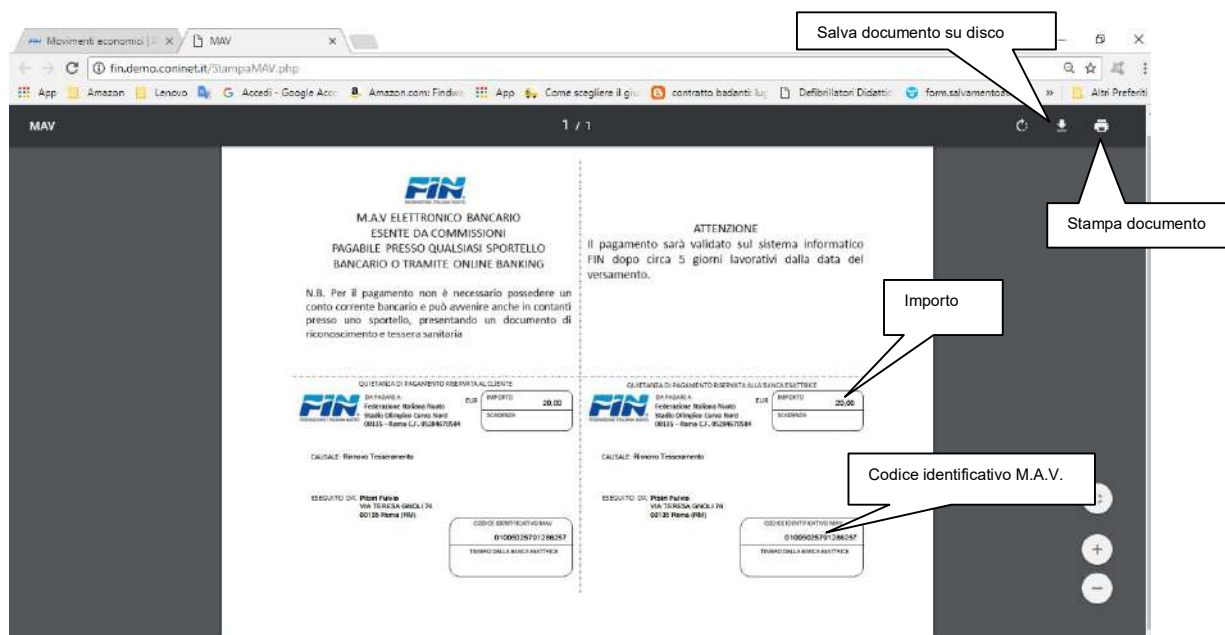
Figura 31:Modello M.A.V.
