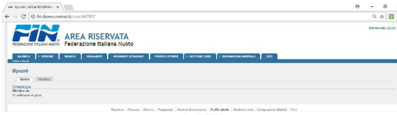
Figura 32: cronologia utente
